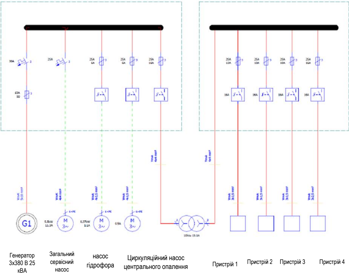
Приклад 1 Розподільний щит 380 В
