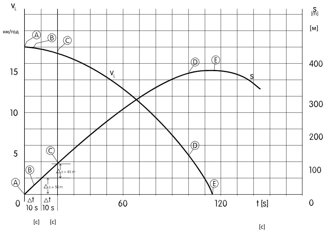
Рисунок 1: Маневр зупинки
