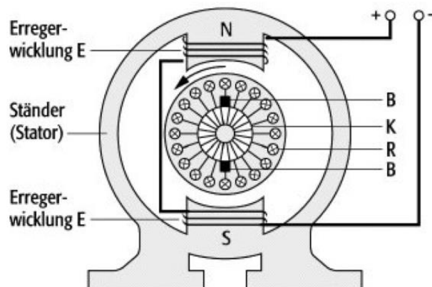
Gleichstrommotor 1: Aufbau; B: Kohlebürsten, R: Rotorwicklung (Läuferwicklung), K: Kommutator (Kollektor, Stromwender).
