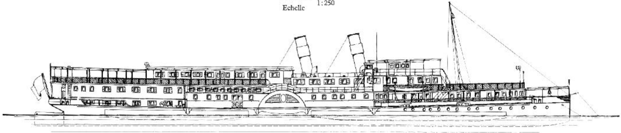
СХЕМА ПАССАЖИРСКОГО СУДНА „ФЕЛСАБАДУЛАШ”
