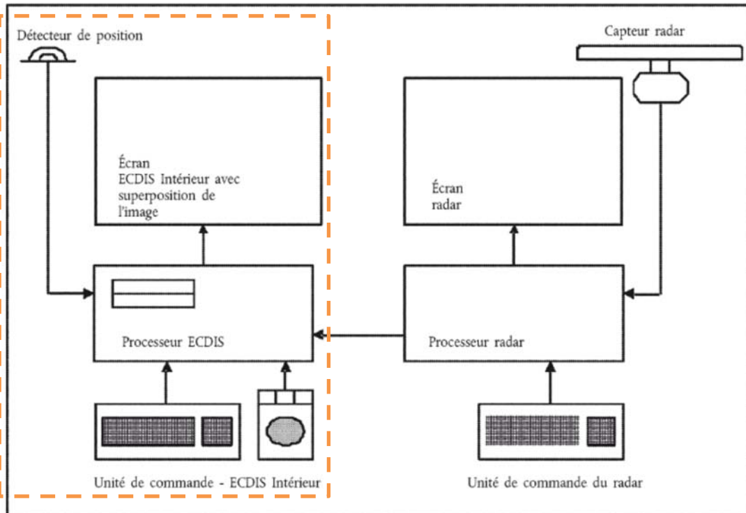
Figure 1 : Appareil ECDIS Intérieur, appareil autonome relié à l'installation radar (configuration du système 2)
