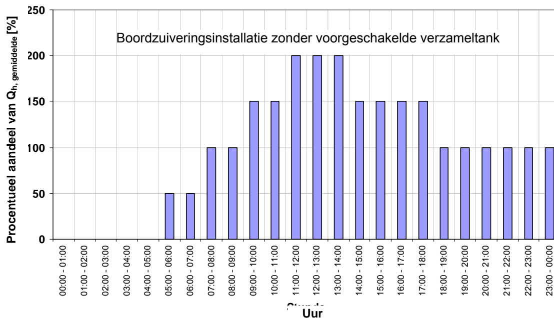
Figuur 2: Dagelijks lineair verloop van de boordzuiveringsinstallatie zonder voorgeschakelde verzameltek van het afvalwater
